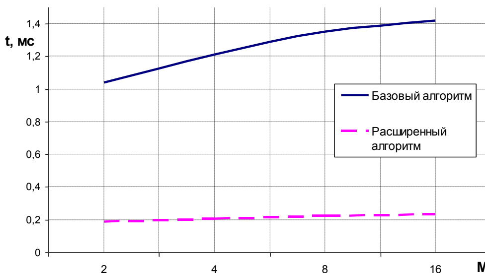
Рис. 5. Результаты экспериментального исследования зависимости времени выполнения микширования t от количество последовательностей M
