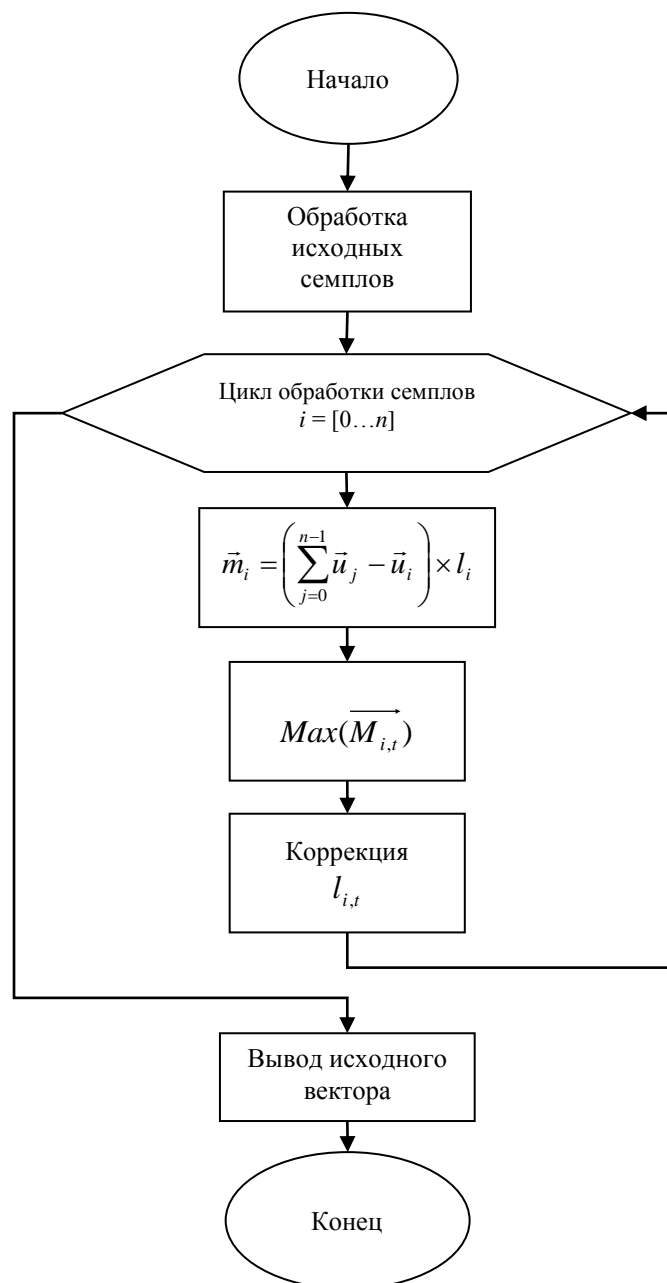
Рис. 2. Блок-схема расширенного алгоритма микширования
