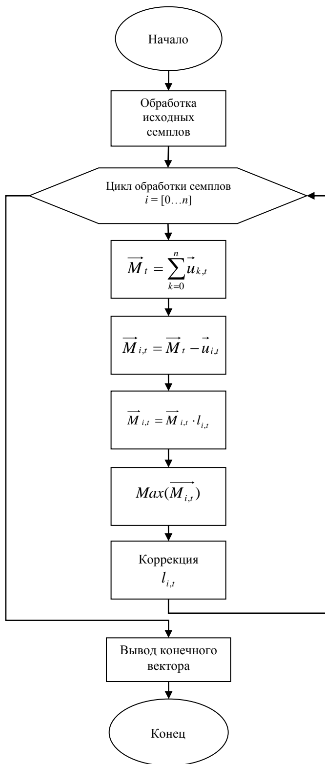
Рис. 1. Блок-схема базового алгоритма микширования
