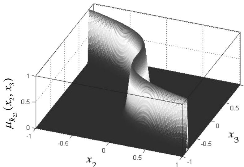
Рис. 4. Вид нечеткого отношения \tilde{R}_{23}
