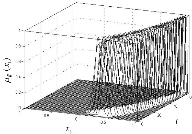
Рис. 7. Нечеткие значения концепта K_1 на 64 эпохах моделирования
