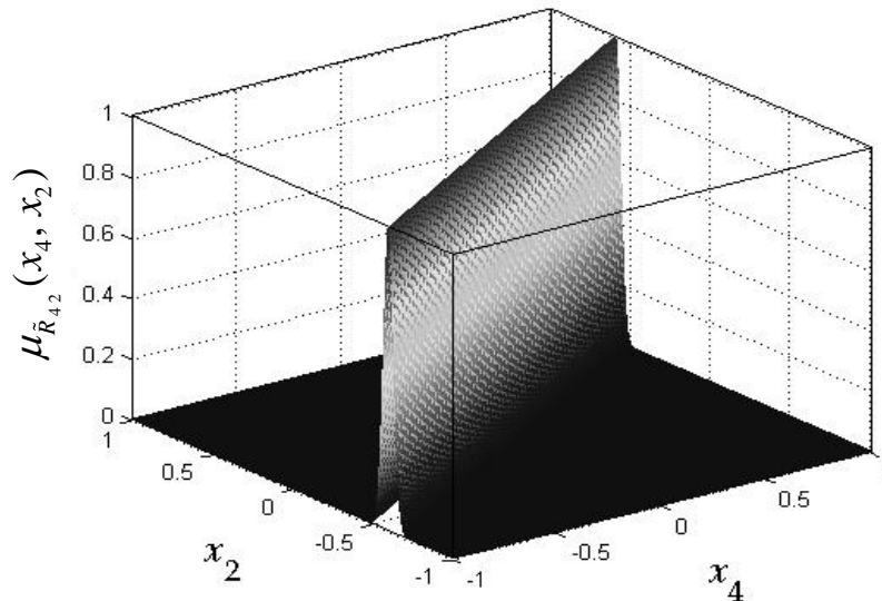
Рис. 2. Пример нечеткого отношения \tilde{R}_{42} между концептами K_4 и K_2
