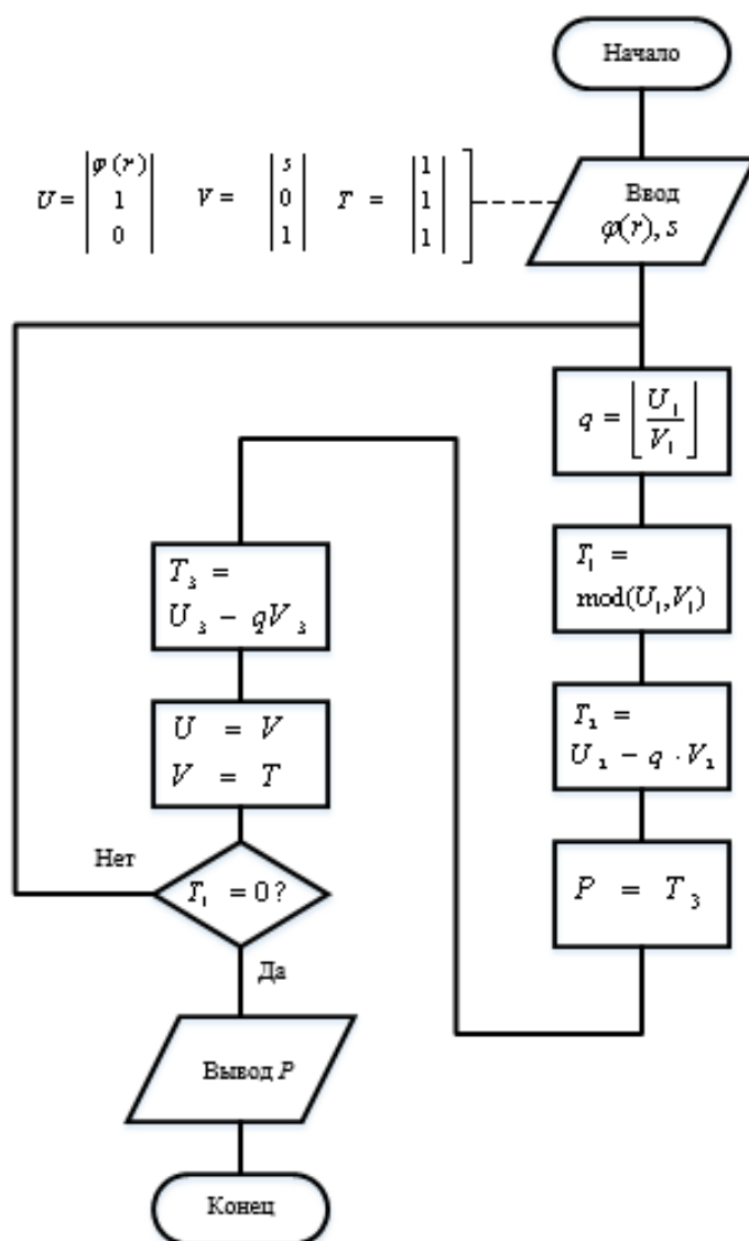
Рис. 1. Обобщённый алгоритм Евклида
