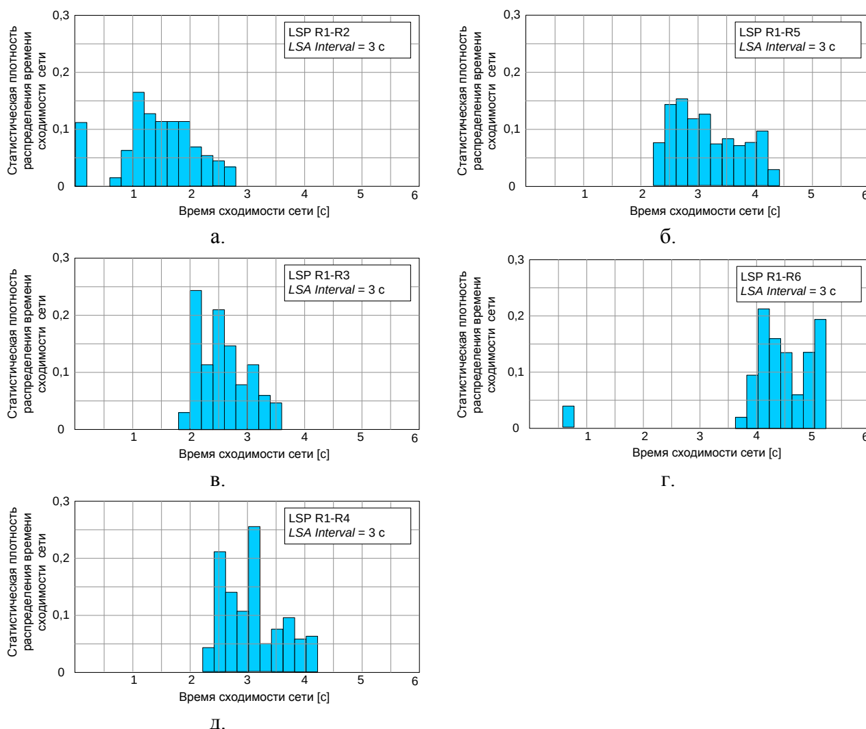
Рис. 22. Распределение статистических оценок времени сходимости при первоначальном установлении путей LSP в сети OSPF-TE [70]
