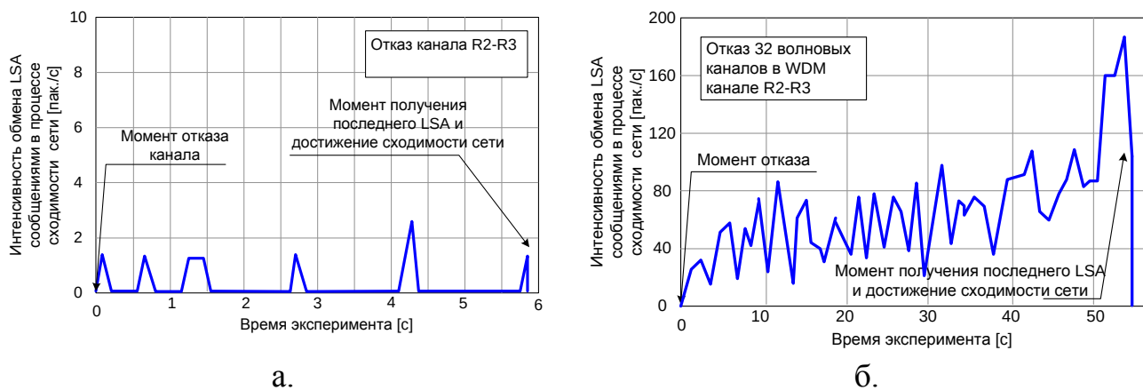
Рис. 24. Интенсивность распространения LSA сообщений, порождаемых отказами в канале связи, для случаев отказа канала связи (а) и отказа подканалов отдельных длин волн в WDM-канале (б) [70]
